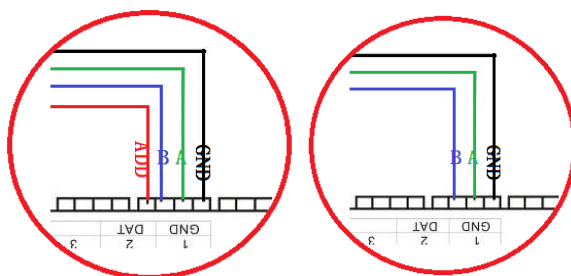
②. DMX512 差分信号线接线图
